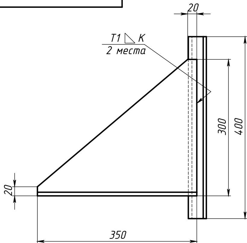
Поз.1 (Основание)
