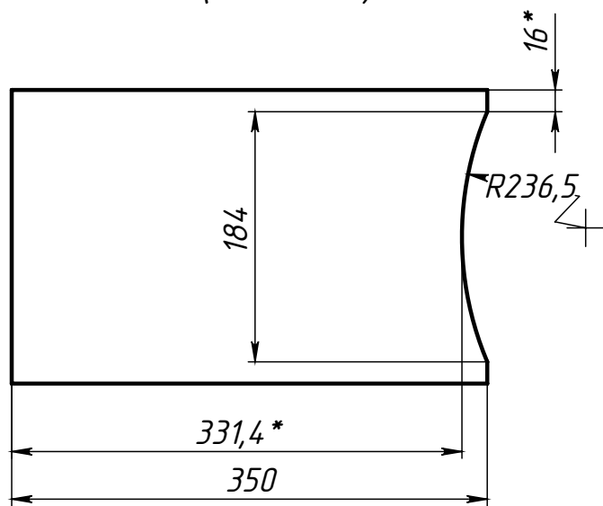
Поз.1 (Основание)
